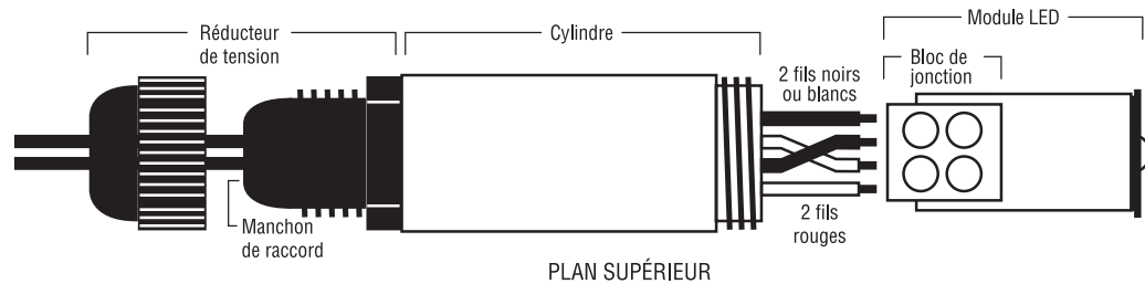
PLAN SUPÉRIEUR
